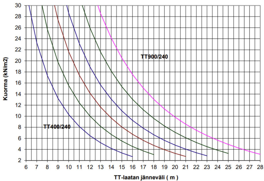
TT3500-240 - C40/50 Tasainen kuorma
