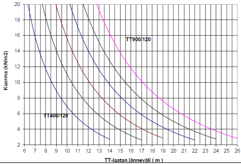
TT3500-170 - C40/50 Tasainen kuorma
